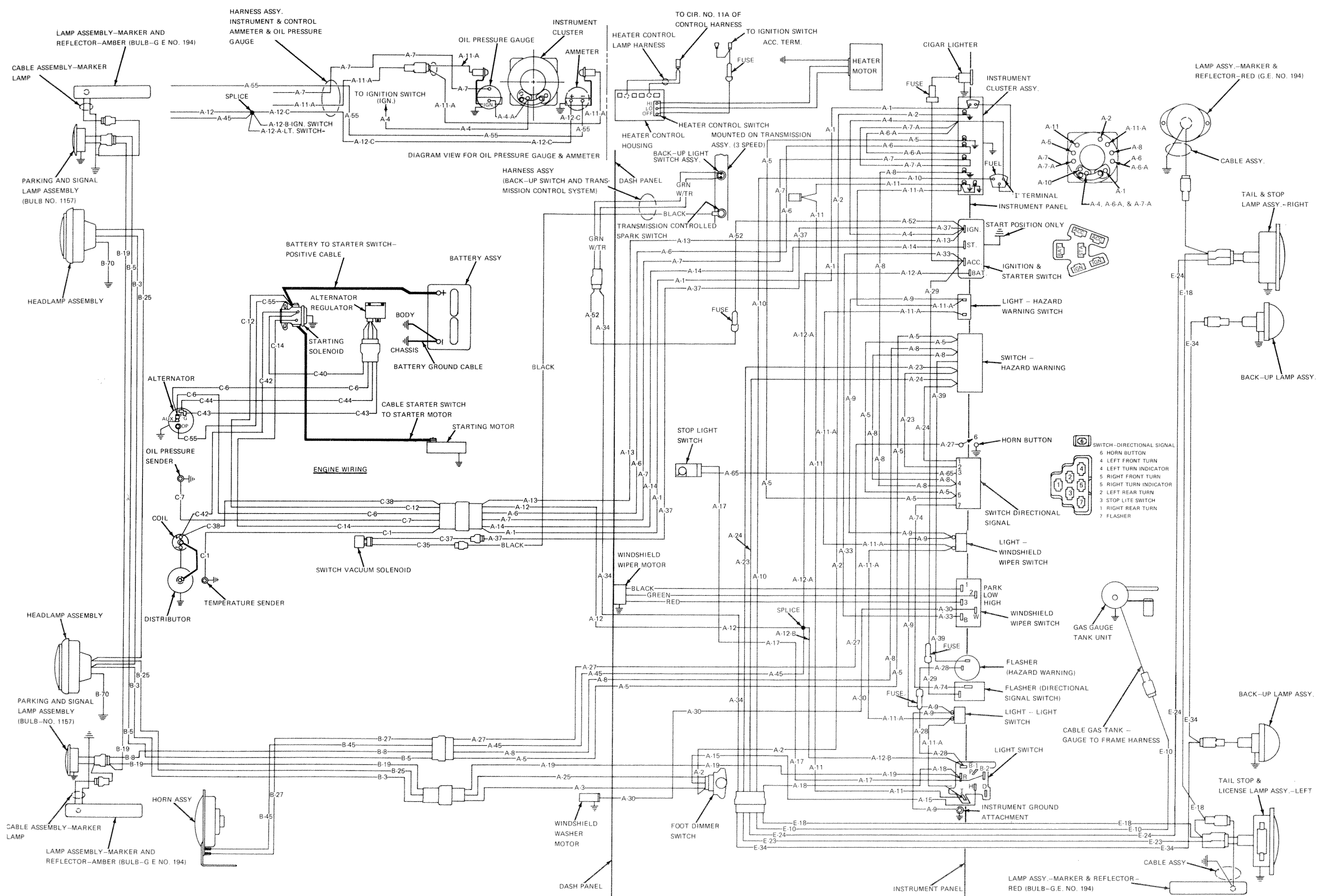
WIRING DIAGRAM-CJ
