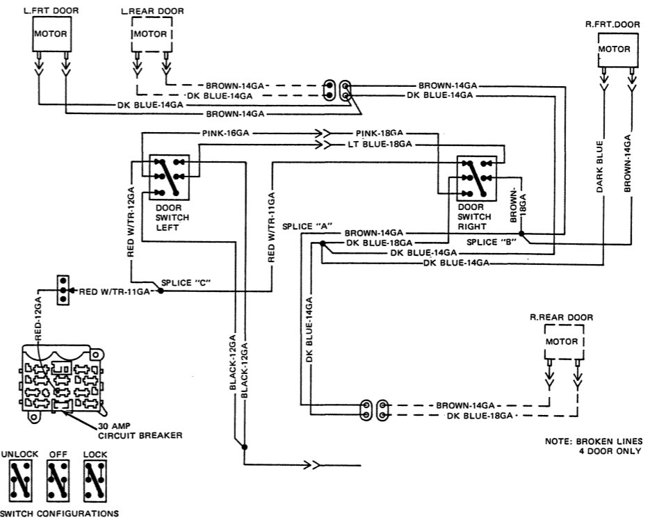
Jeep Power Door Locks 4 Door
