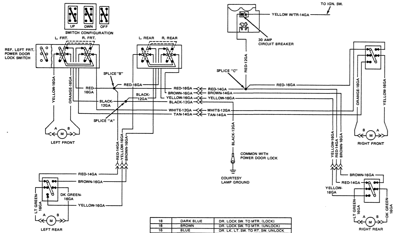
Jeep Power Windows 4 Door
