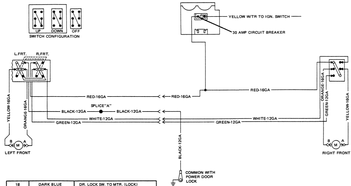
Jeep Power Windows 2 Door
